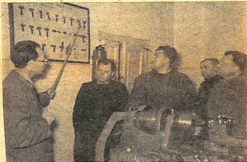
На фото: викладач інституту тов. Чумак пояснює вчителям шкіл Київської області обробку металу на токарних верстатах за допомогою різноманітних різців.
